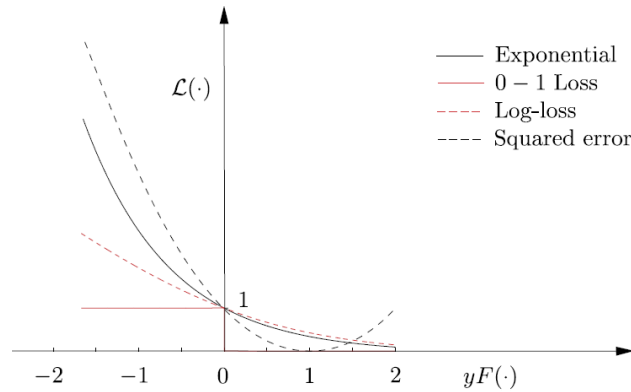
Figura 8-2: Comparação de diferentes funções de loss (retirado de [8]).
